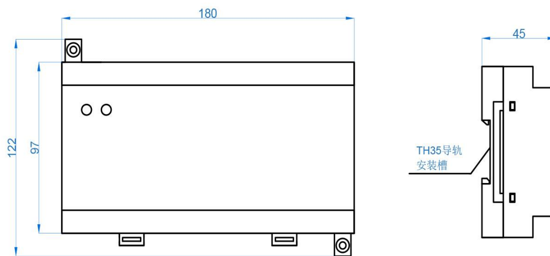
A3、A24、A48模块的外形尺寸
