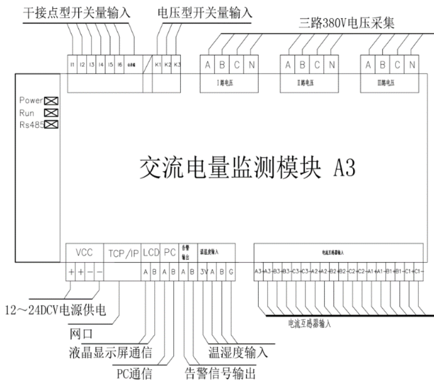
A3模块接线图
