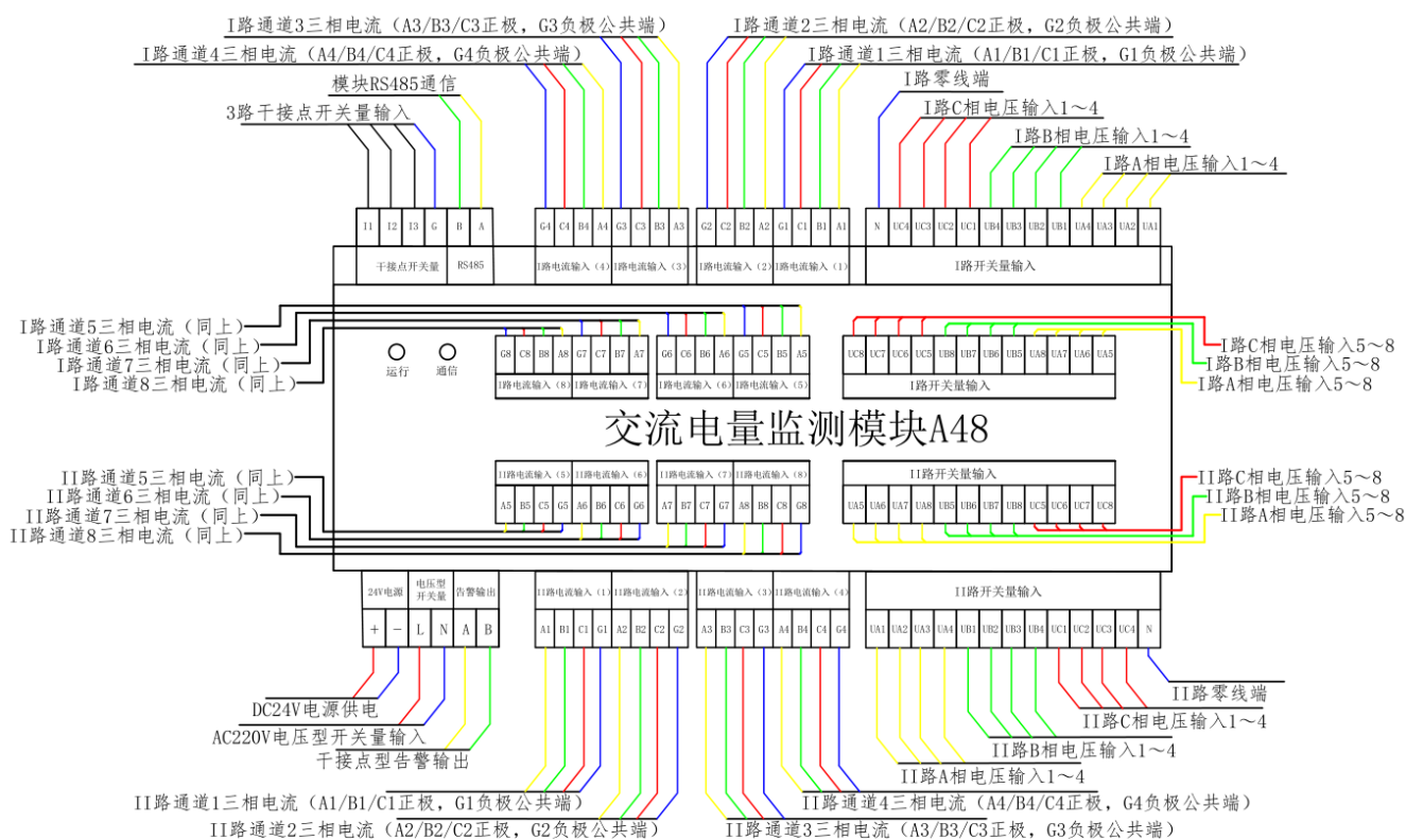
A48模块接线图
