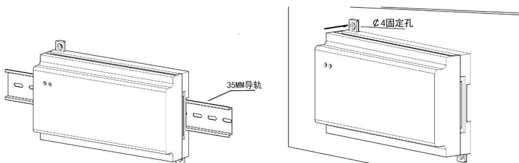
模块安装图（导轨式）
