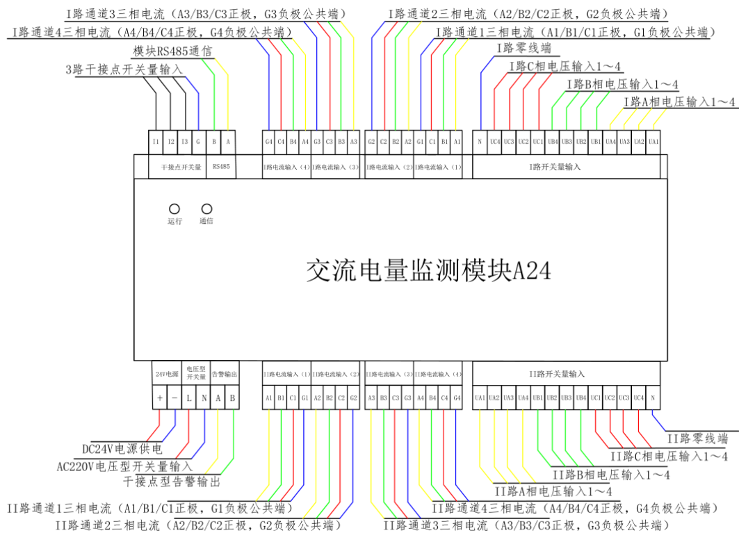
A24模块接线图
