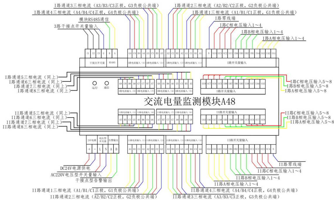
A48模块接线图
