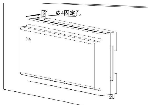
模块安装图（面板式）
