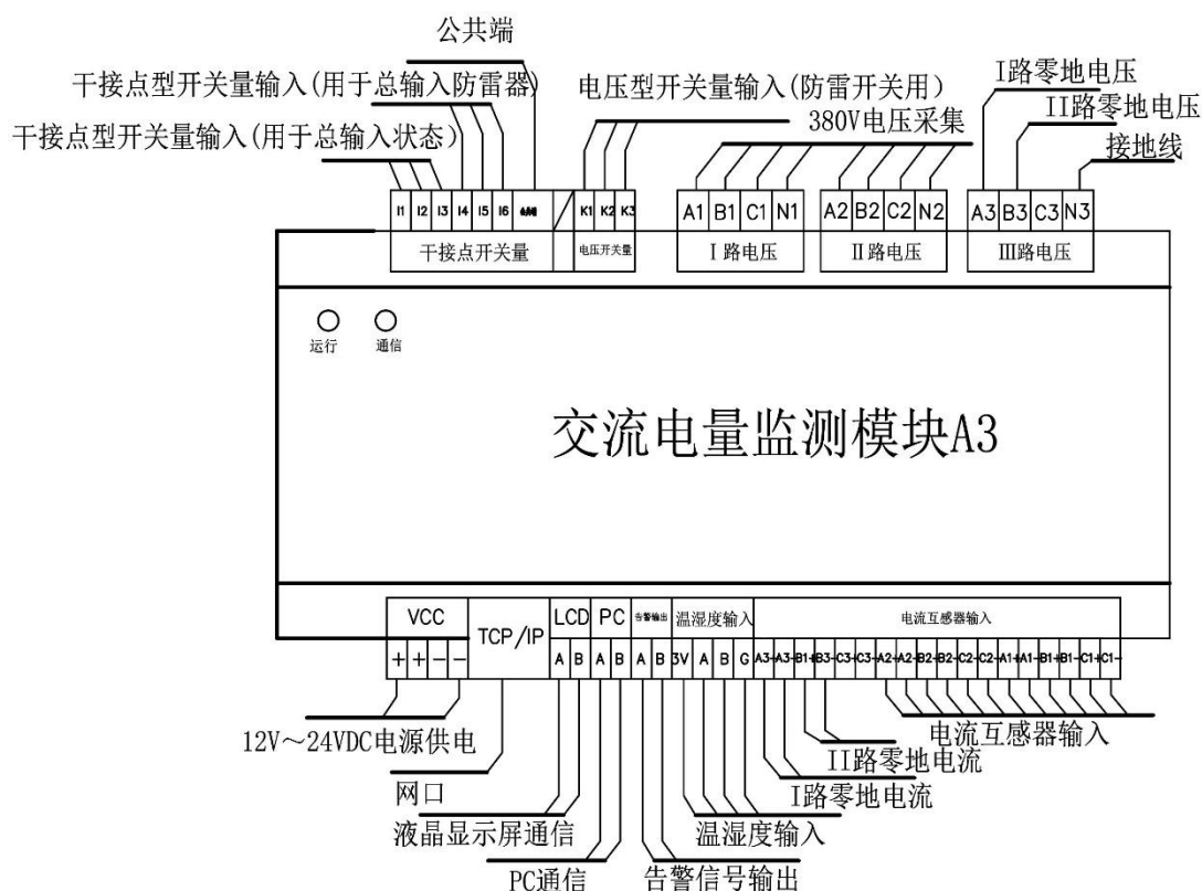
A3模块2路三相进线加零线监测接线图
