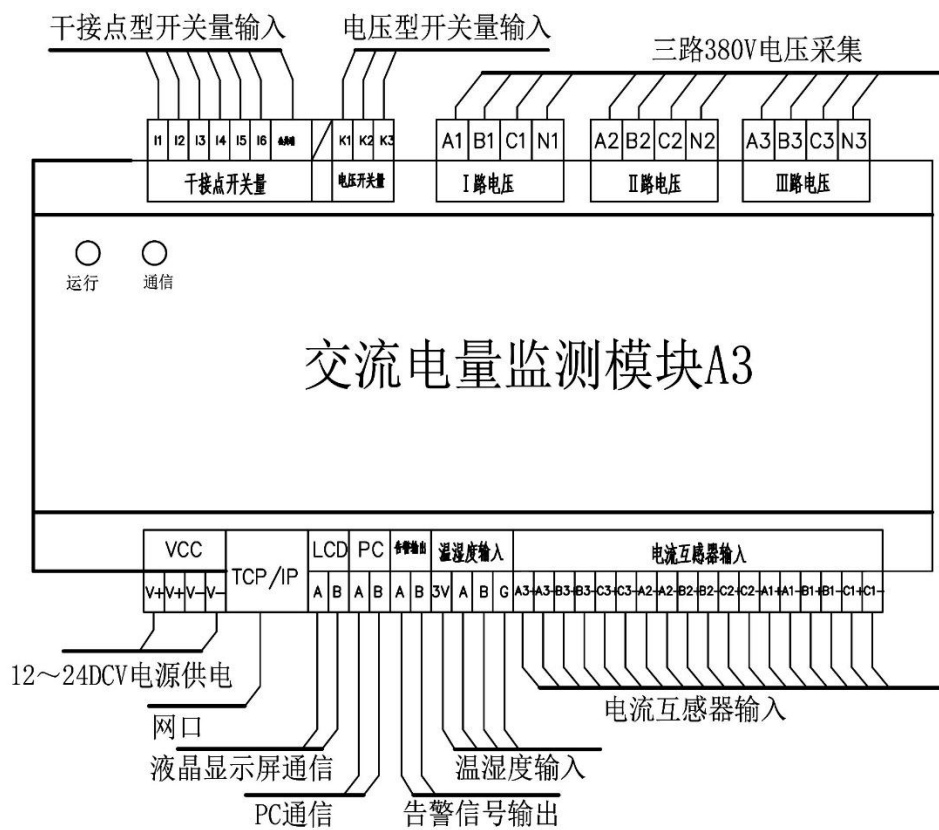
A3模块3路三相进线接线图
