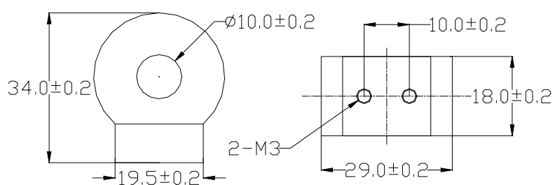
CT09系列电流互感器外形尺寸图
